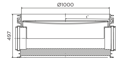
Inlet/outlet DN250
