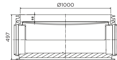
Inlet/outlet DN315
